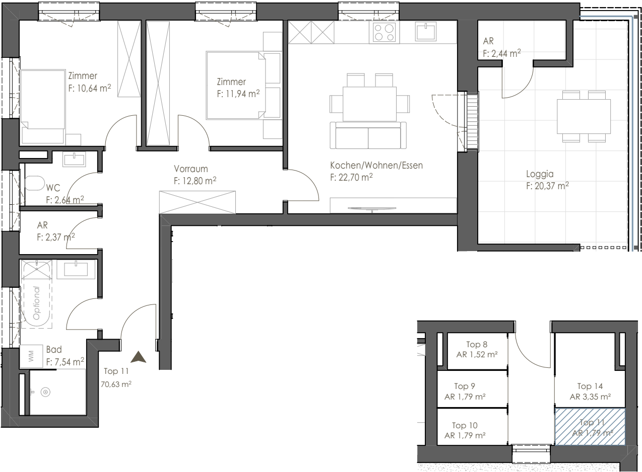
Wohnungsgrundriss 1.Obergeschoß
