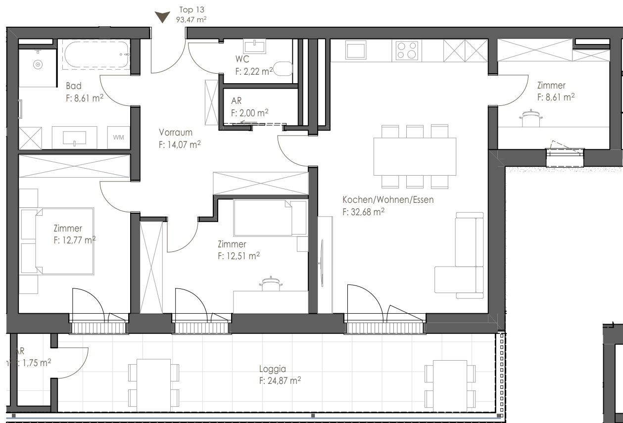
Wohnungsgrundriss 2.Obergeschoß
