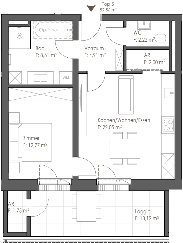
Wohnungsgrundriss 1.Obergeschoß
