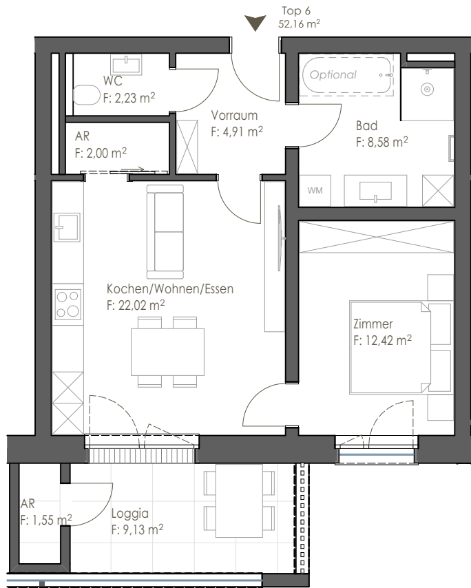
Wohnungsgrundriss 1.Obergeschoß
