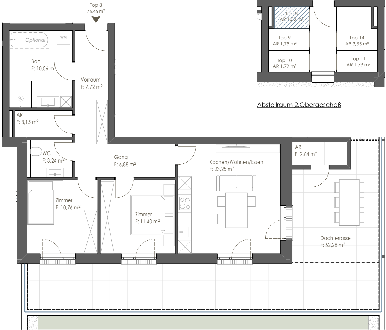
Wohnungsgrundriss 1.Obergeschoß
