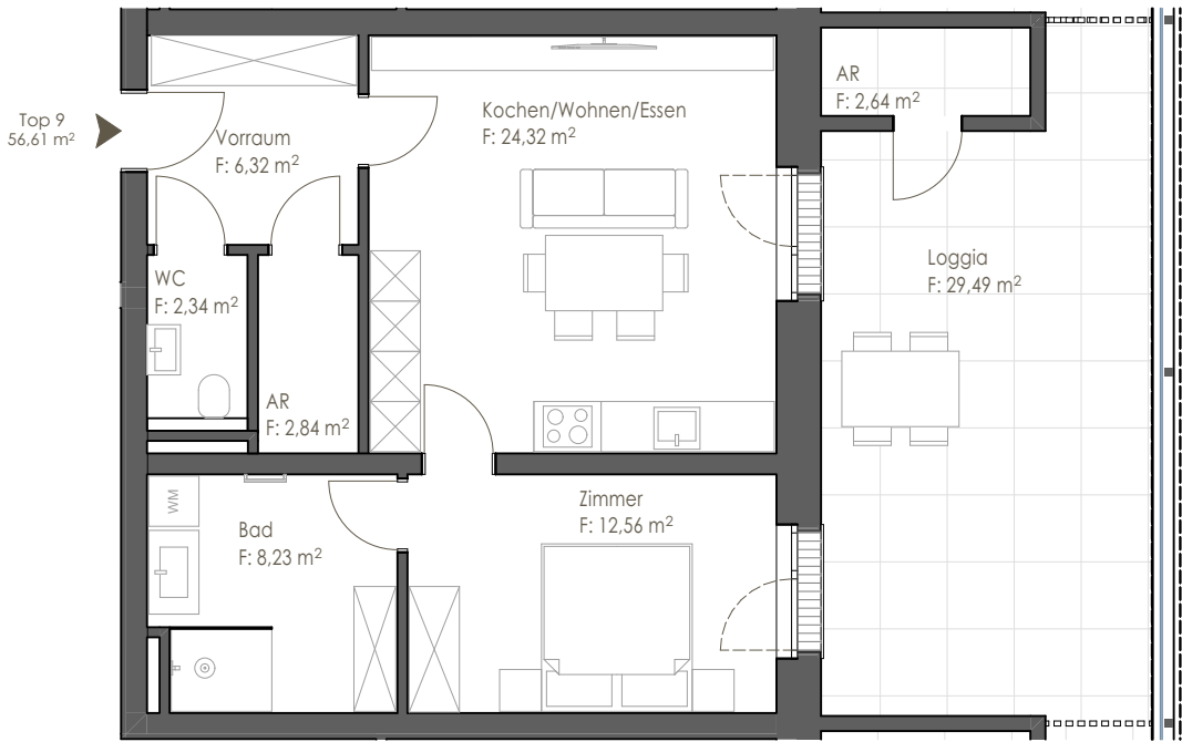
Wohnungsgrundriss 1.Obergeschoß
